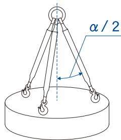
3点吊り
