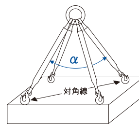
4点吊り
